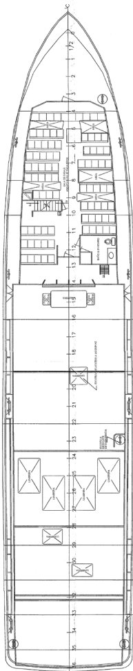
CUBIERTA PRINCIPAL 4.05 m SOBRE LB.
