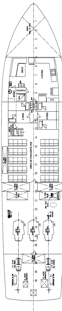
BAJO CUBIERTA
